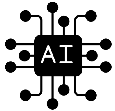
AI & ML
